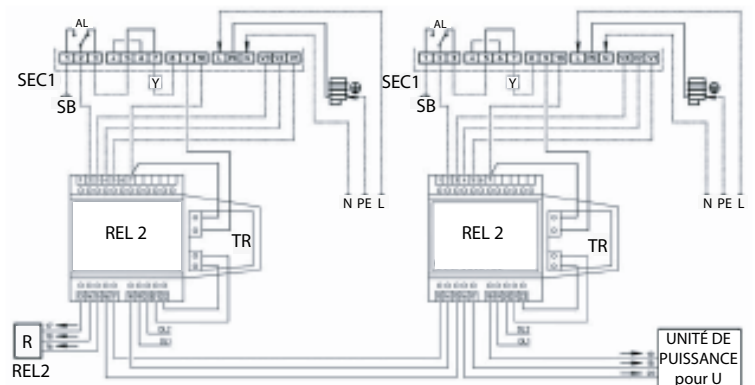
Schéma 8 - Raccordement REL02 avec 1 vanne
