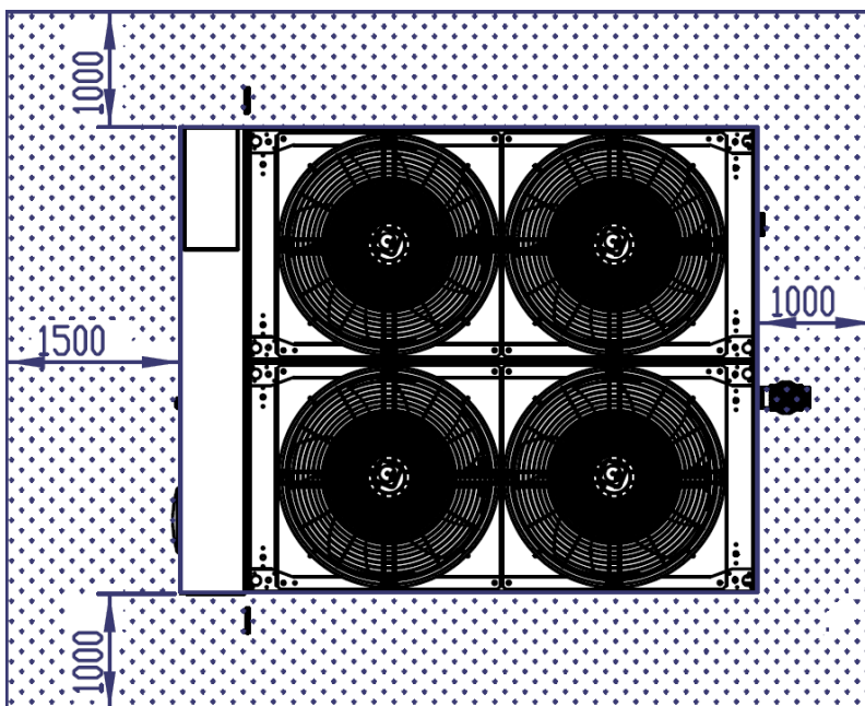
Schéma 4b Dégradations minimum [mm] pour une unité 2 V
