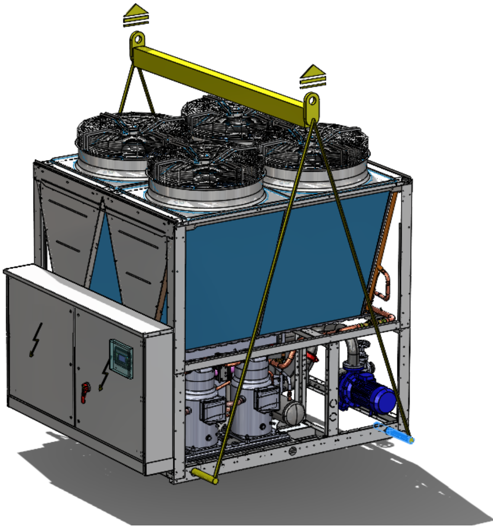
Schéma1a Procédure de levage correcte Version 2 V
