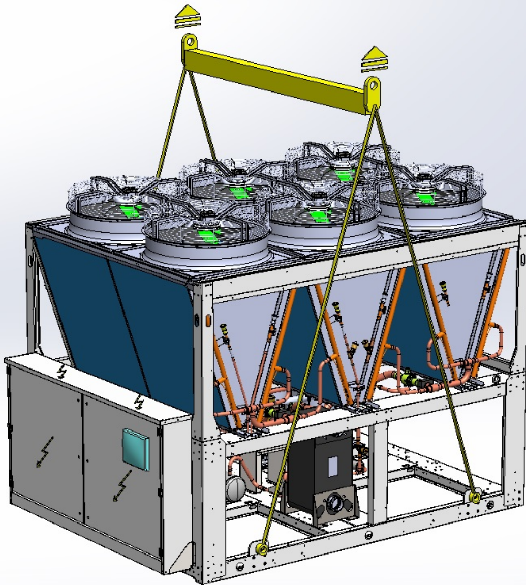
Schéma 2b Procédure de levage correcte Version 3 V
