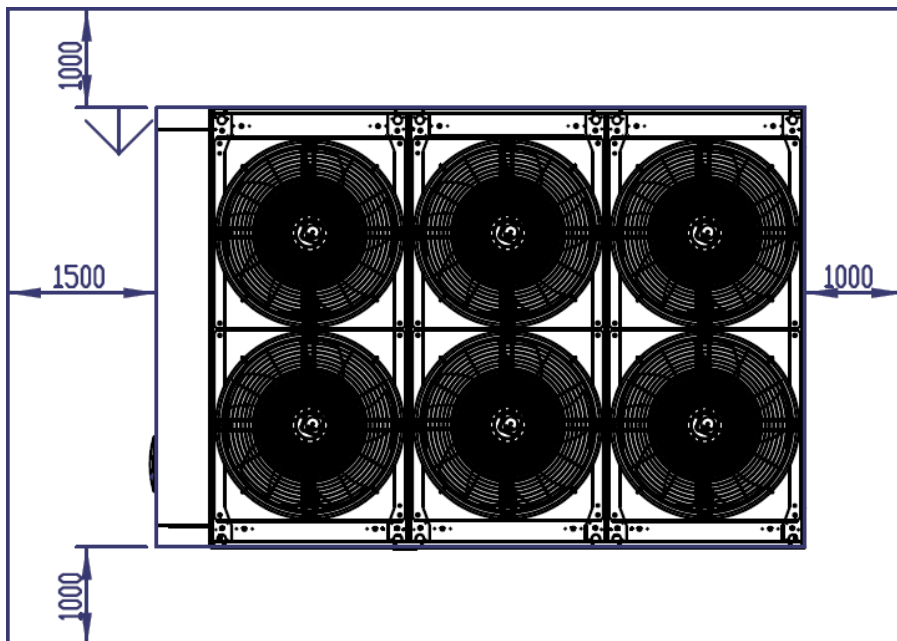
Schéma 5c Dégagements minimum requis [mm] pour une unité 3 V
