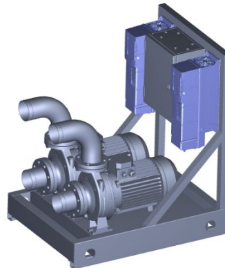
2 x Einzelpumpen- Hydraulikmodul mit oder ohne Umrichter
