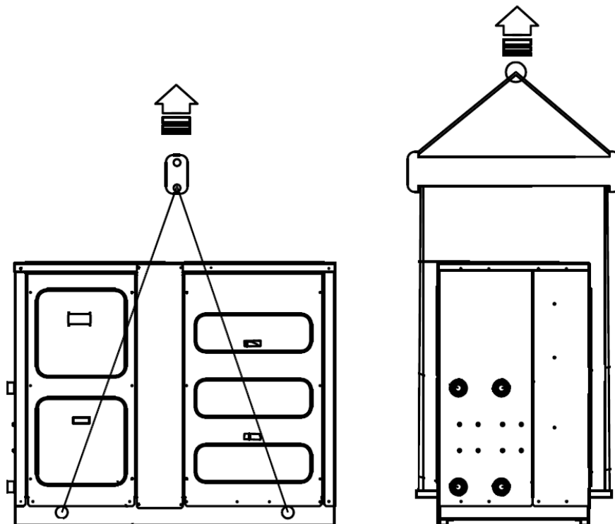
Abbildung 2 – Richtiger Hebevorgang für Plattform 1-Einheiten (CGWF SE-Größen von 050 bis 090 – CGWF HE-Größen von 055 bis 095 – CXWF Größen von 060 bis 110)
