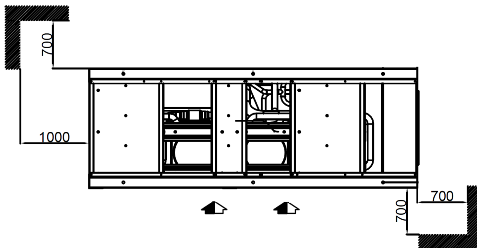
Abbildung 8 - Minimaler Platzbedarf [mm] für Plattform 1-Einheiten (Größen mit zwei Kältemittelkreisläufen - CGWF SE-Größen von 115 bis 475, CGWF HE-Größen von 115 bis 500 und CXWF-Größen von 130 bis 565)
