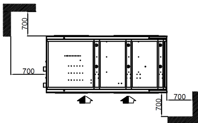
Abbildung 7 – Minimaler Platzbedarf [mm] für Plattform 2-Geräte (Korrektes Hebeverfahren für Geräte mit Rahmen der Größe 2 (CGWF SE-Größen von 110 bis 150 – CGWF HE-Größen von 110 bis 155 – CXWF-Größen von 125 bis 175))
