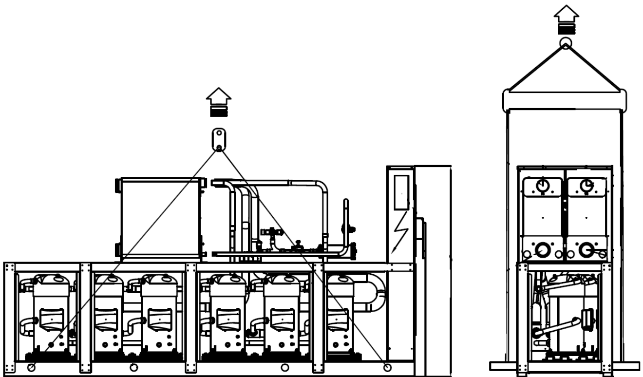
Abbildung Richtiger Hebevorgang für Plattform 4-Einheiten (Größen mit zwei Kältemittelkreisläufen - CGWF SE-Größen von 555 bis 700, CGWF HE-Größen von 585 bis 700 und CXWF-Größen von 670 bis 835)
