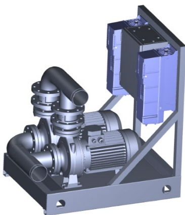
Einzelpumpen- Hydraulikmodul mit oder ohne Umrichter
