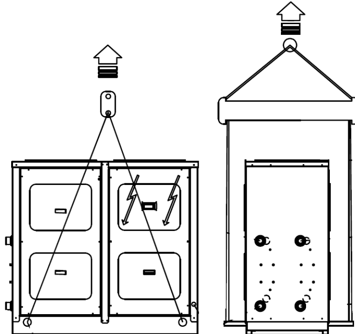
Abbildung 2 – Richtiger Hebevorgang für Plattform 1-Einheiten (CGWF SE-Größen von 050 bis 090 – CGWF HE-Größen von 055 bis 095 – CXWF Größen von 060 bis 110)
