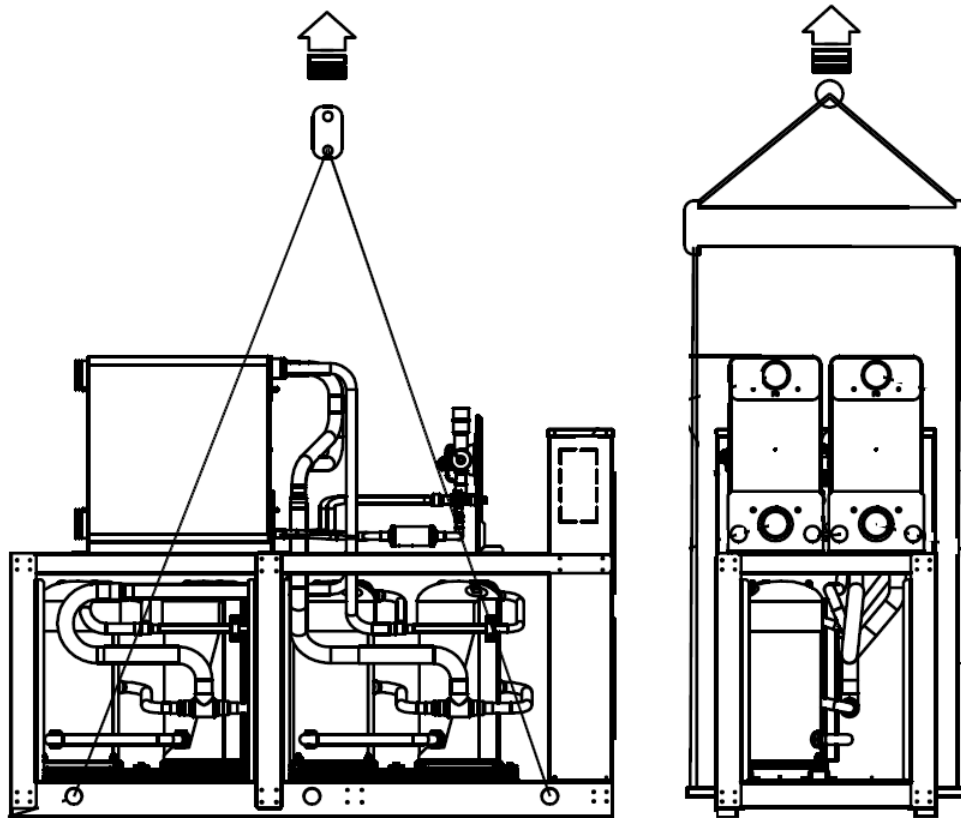
Abbildung 4 Richtiger Hebevorgang für Plattform 3-Einheiten (Größen mit zwei Kältemittelkreisläufen - CGWF SE-Größen von 115 bis 475, CGWF HE-Größen von 115 bis 500 und CXWF-Größen von 130 bis 565)
