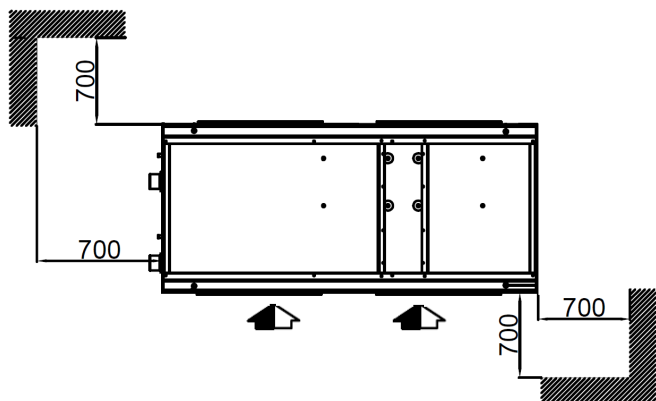
Abbildung 6 – Minimaler Platzbedarf [mm] für Plattform 1-Einheiten (CGWF SE-Größen von 050 bis 090 – CGWF HE-Größen von 055 bis 095 – CXWF-Größen von 060 bis
