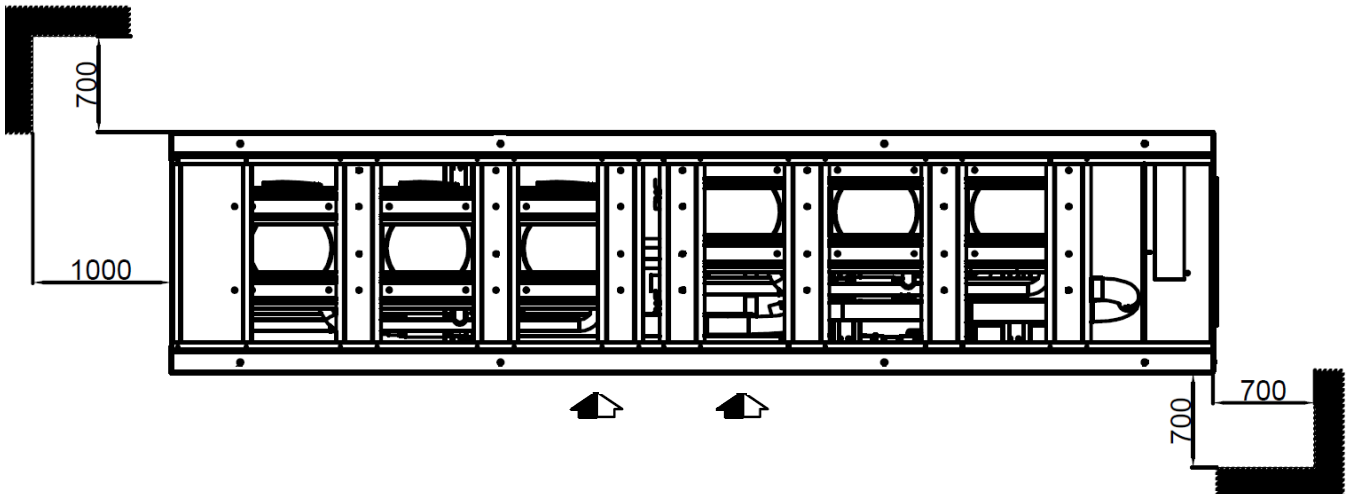
Abbildung 9 - Minimaler Platzbedarf [mm] für Plattform 4 Einheiten (Größen mit zwei Kältemittelkreisläufen - CGWF SE-Größen von 555 bis 700, CGWF HE- Größen von 585 bis 700 und CXWF-Größen von 670
